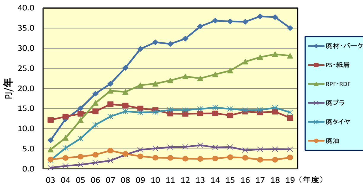
図 6 バイオマス・廃棄物使用量の推移
