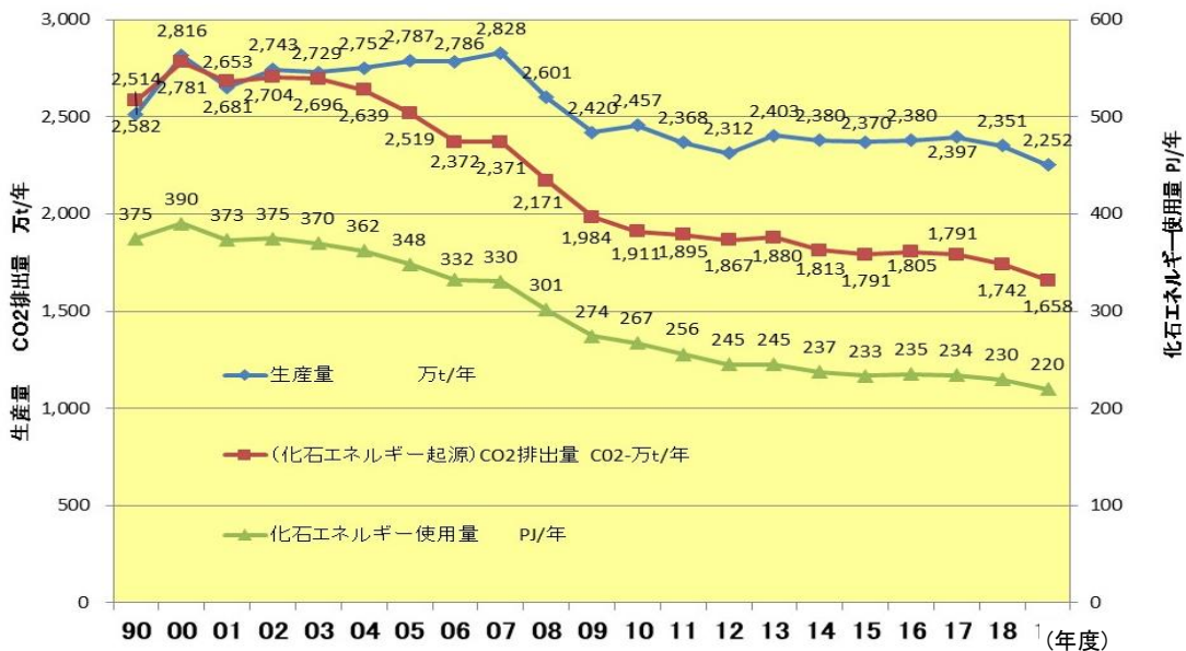
図1 生産量とCO 2 排出量及び化石エネルギー使用量の推移
