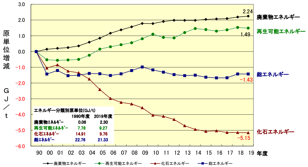
図3 エネルギー分類別原単位の推移 (GJ/t 1990年度基準)
